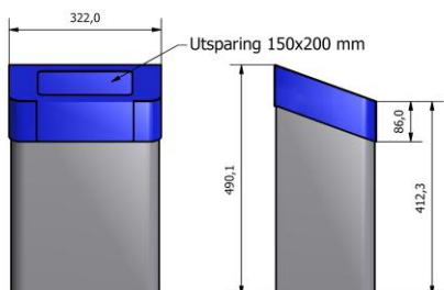
Skrå sekkeskjuler redusert innkast (art.nr: 290611)
